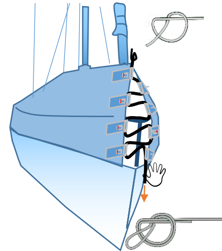
Piano sluiting
